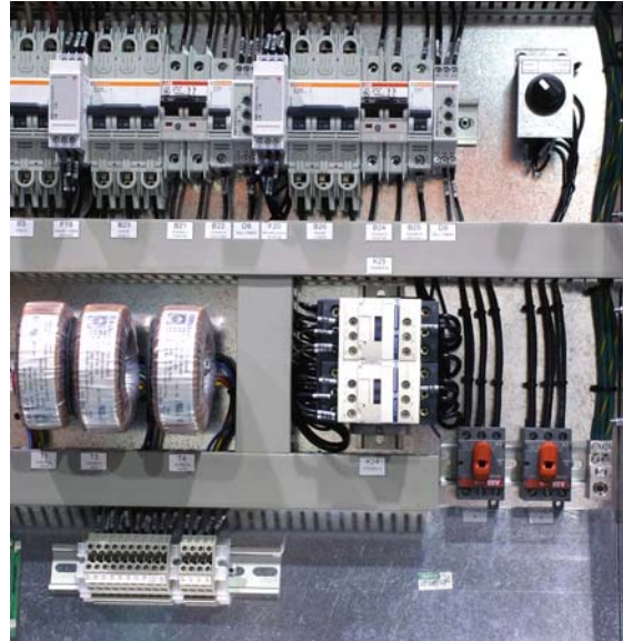
Panneau d'alimentation ClimateWorx comprenant les composants du commutateur convertisseur automatique et du commutateur de sélection d'alimentation électrique
